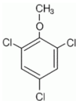
Abbildung 1. 2,4,6-Trichloranisole
